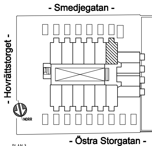
PLAN 3 16 STUDENTLÄGENHETER
